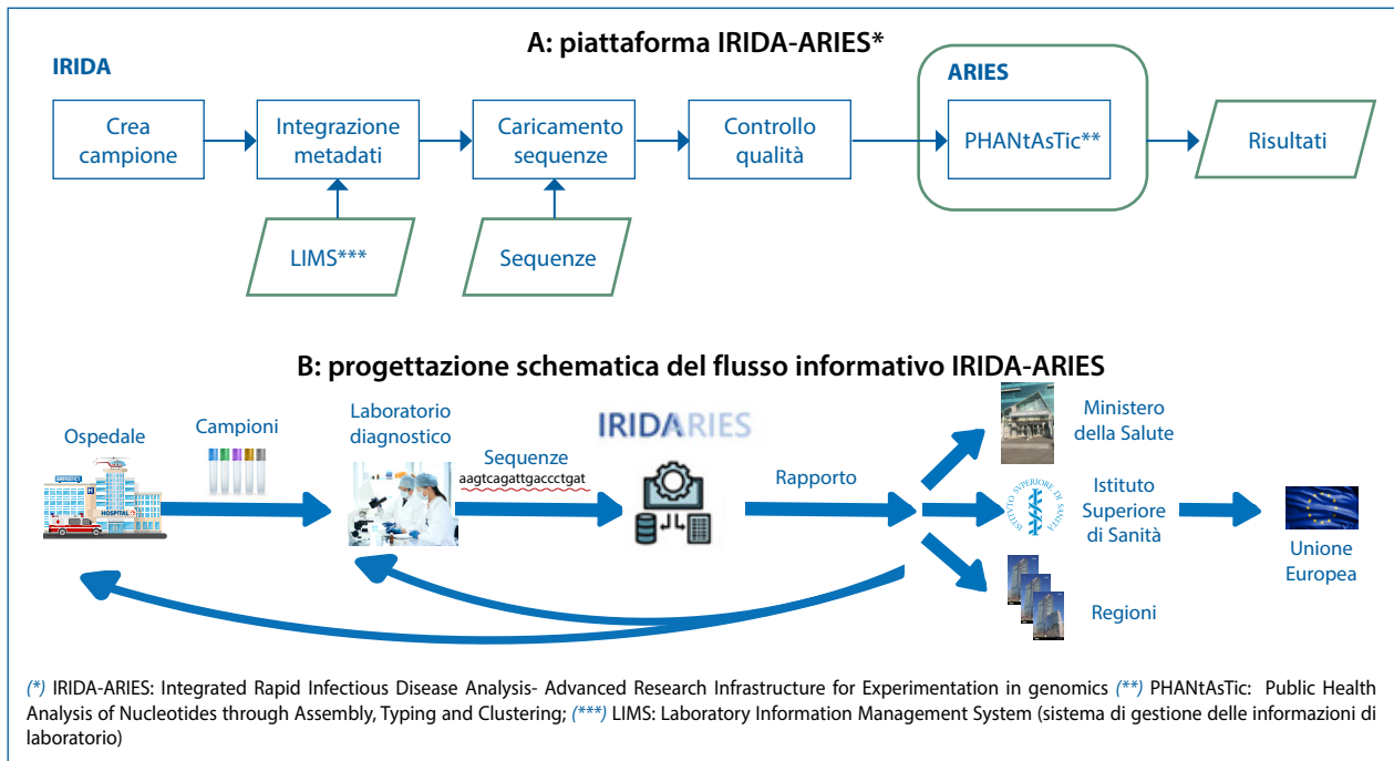
Figura 1 - A: quando si crea un campione, i metadati si recuperano sia dai sistemi informativi di dati molecolari che epidemiologici locali. Quando le sequenze genomiche vengono caricate, si esegue il controllo di qualità e si lanciano le analisi automatiche con la pipeline patogeno-specifica PHANtAsTic. I risultati vengono restituiti a IRIDA e visualizzati in una pagina web. B: il flusso viene attivato a livello locale da un centro che invia un campione di un caso a un laboratorio che esegue il sequenziamento dell'intero genoma. Le sequenze vengono caricate su IRIDA-ARIES e i risultati vengono restituiti a livello locale e inoltrati a livello regionale e nazionale. Se necessario, i dati possono essere portati a livello europeo
